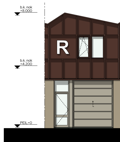
Voorgevel 1:100
