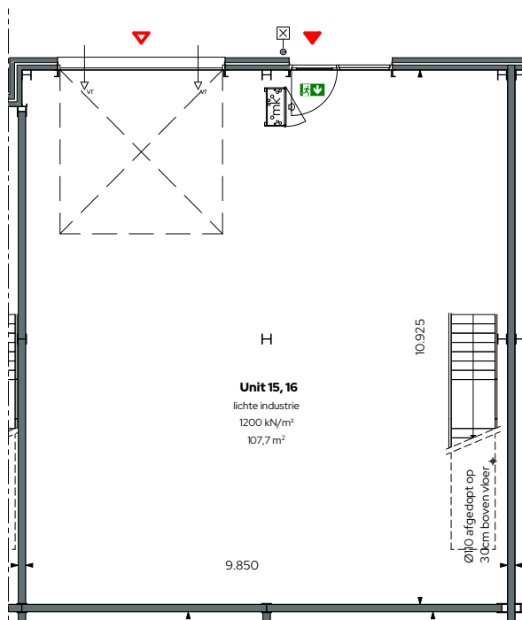
Begane grond 1:100
