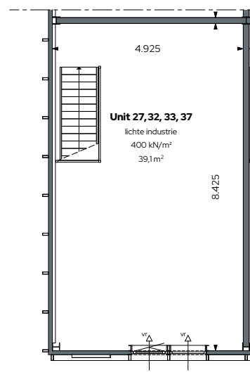
Verdieping 1:100
