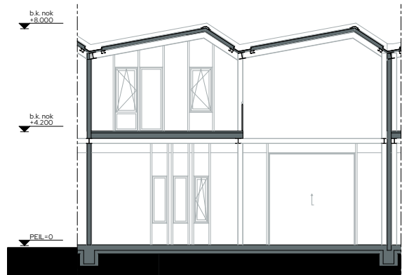
Doorsnede 1:100
