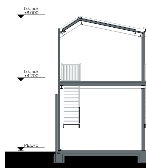
Doorsnede 1:100
