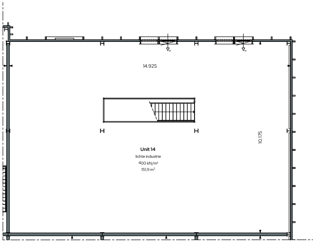
Verdieping 1:100
