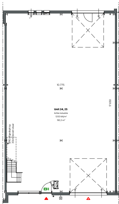
Begane grond 1:100
