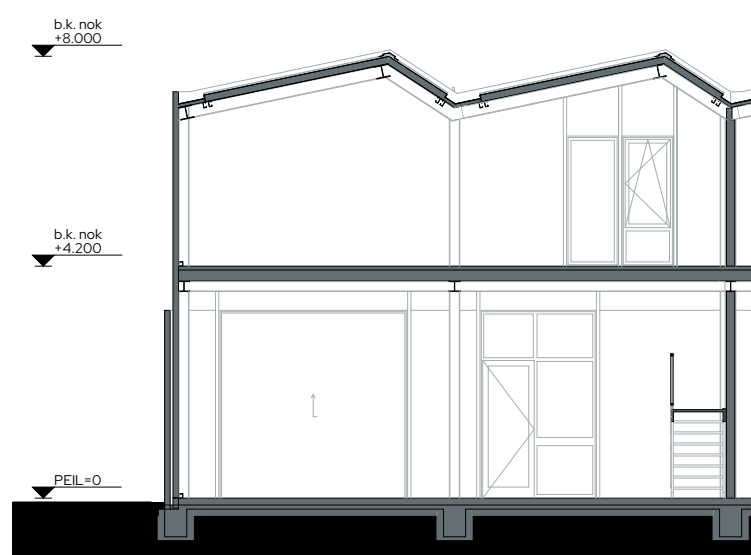
Doorsnede 1:100
