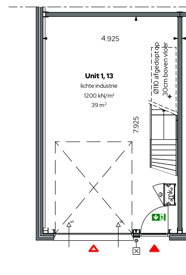
Begane grond 1:100
