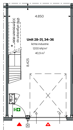
Begane grond 1:100
