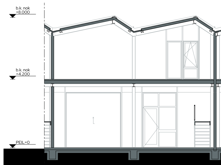
Doorsnede 1:100
