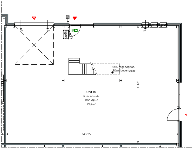
Begane grond 1:100
