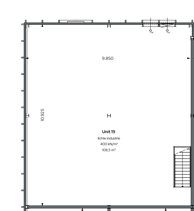
Verdieping 1:100
