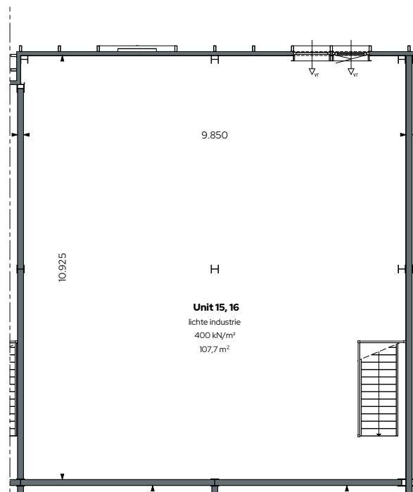
Verdieping 1:100
