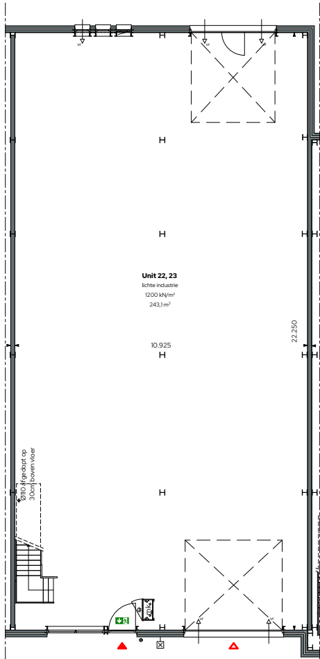
Begane grond 1:100
