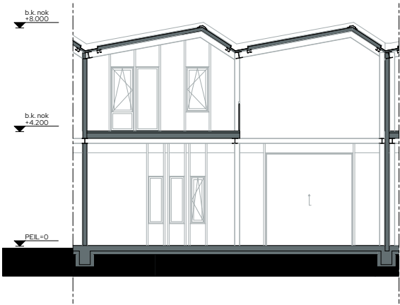
Doorsnede 1:100
