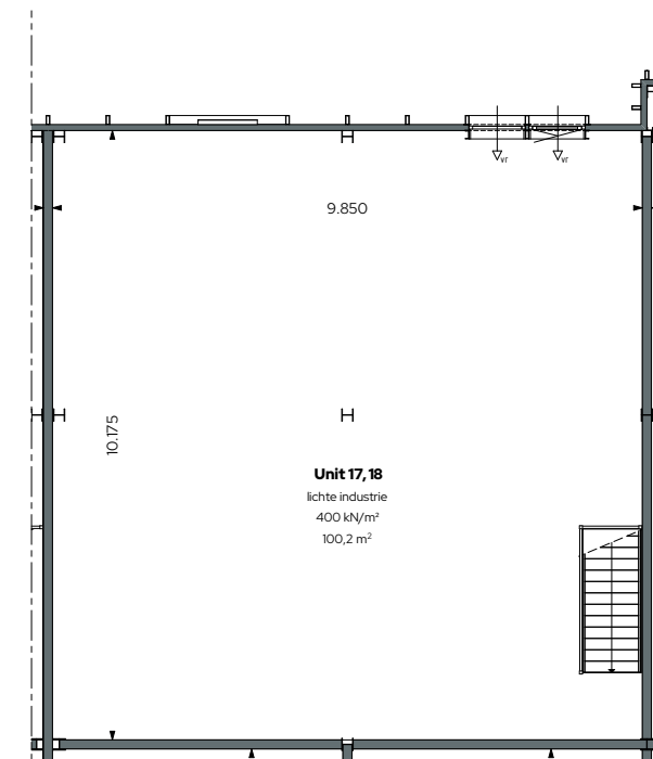
Verdieping 1:100
