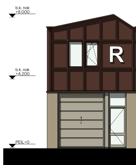
Voorgevel 1:100
