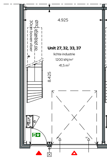
Begane grond 1:100
