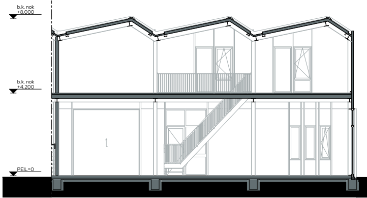
Doorsnede 1:100
