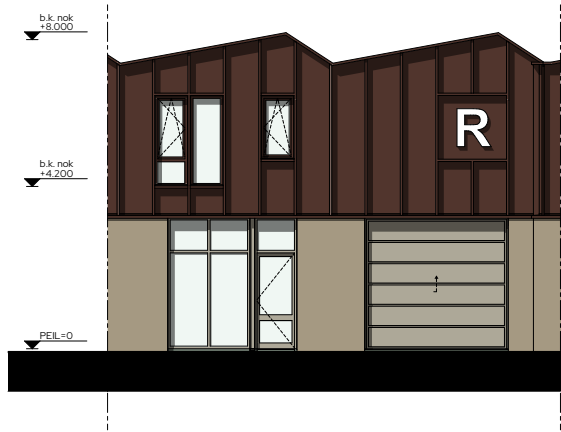
Voorgevel 1:100
