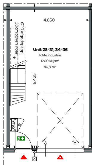
Begane grond 1:100
