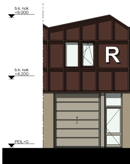
Voorgevel 1:100
