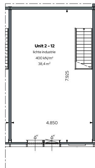
Verdieping 1:100
