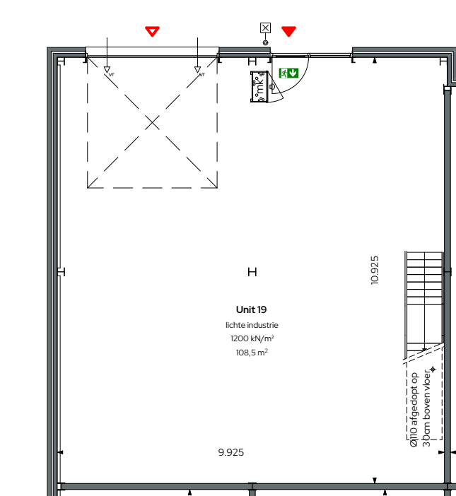
Begane grond 1:100
