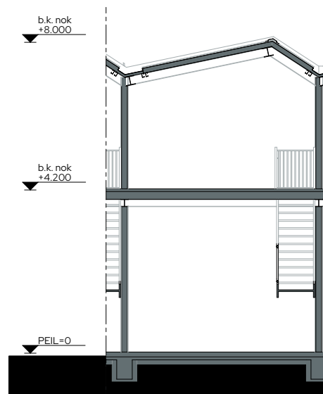
Doorsnede 1:100
